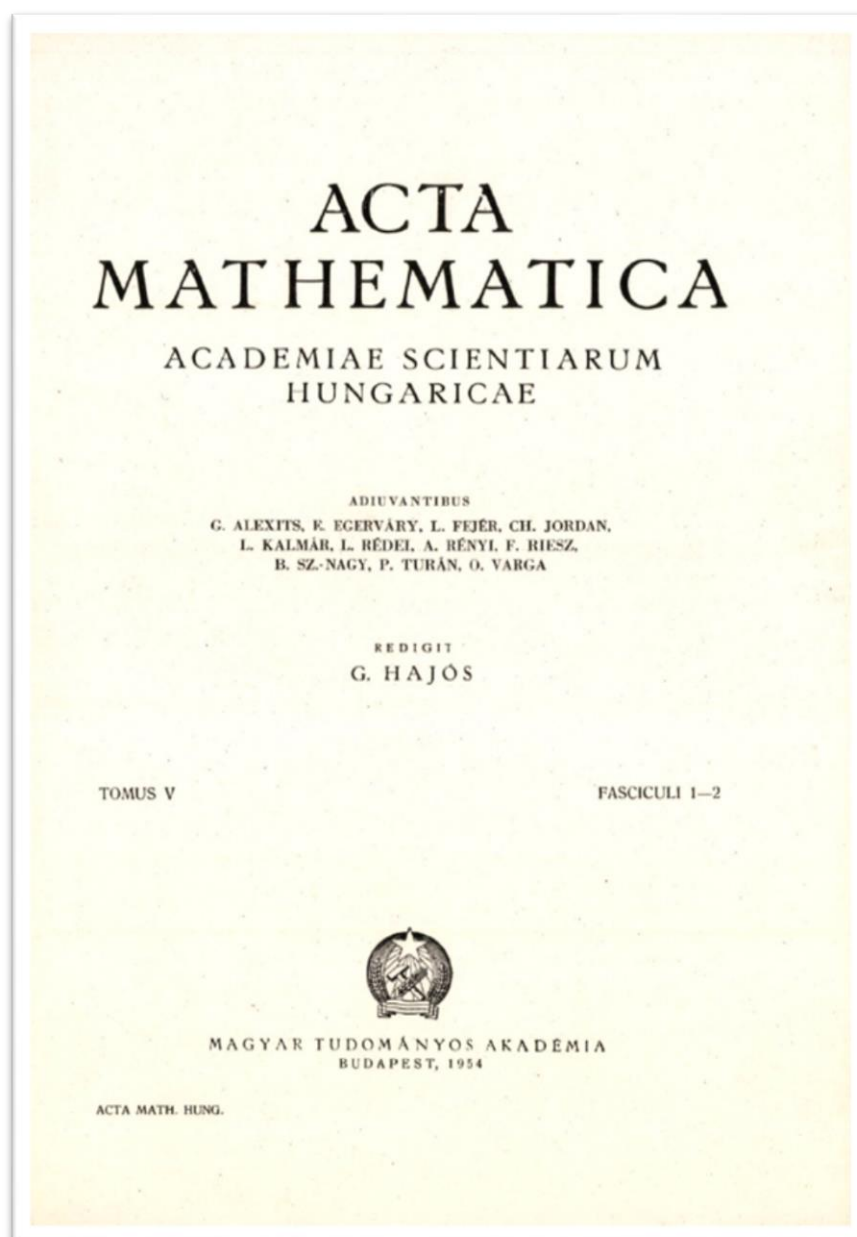
Acta Mathematica Academiae Scientiarum Hungaricae, Tomus 5. (1954)
